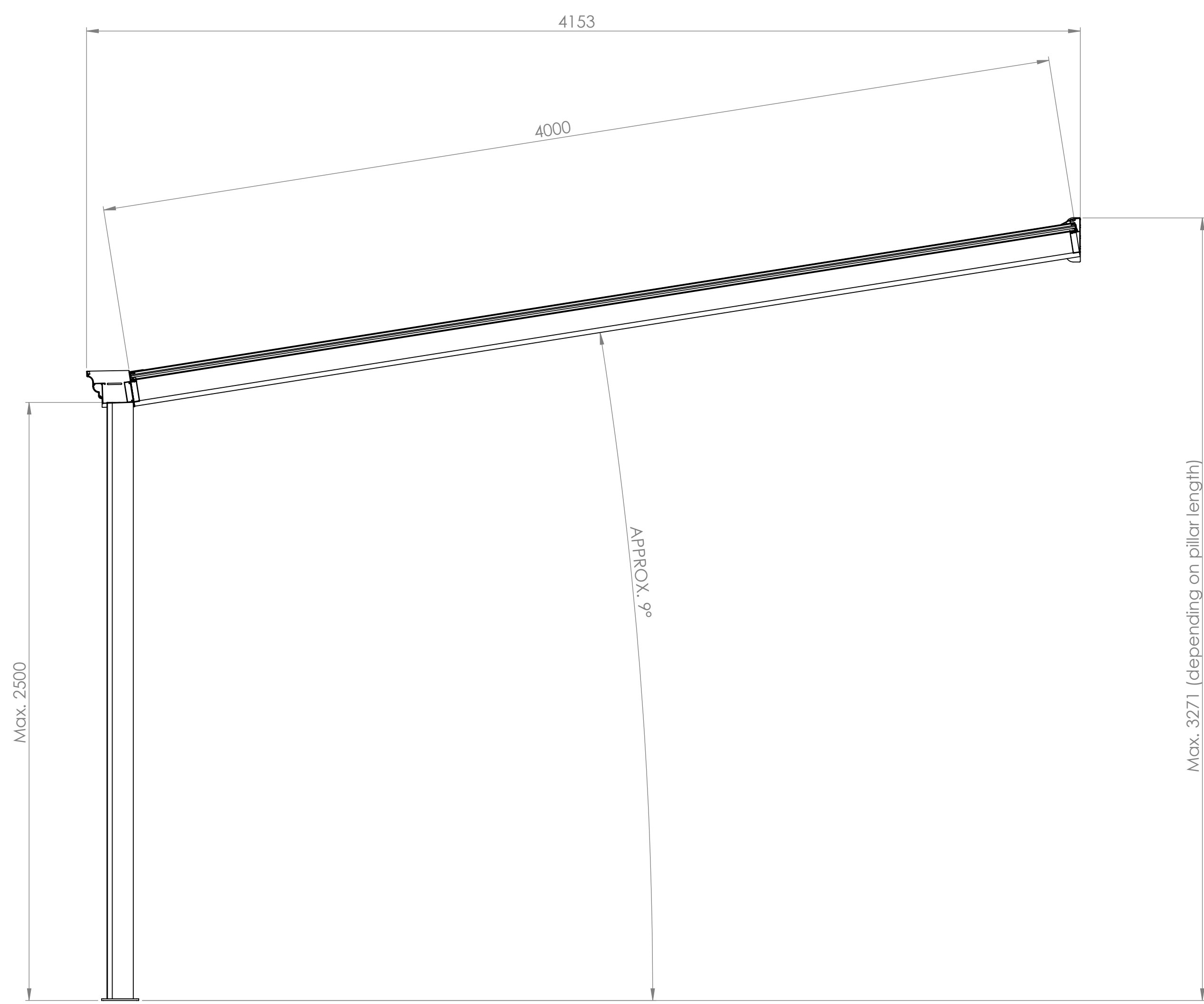
SECTION A-A
